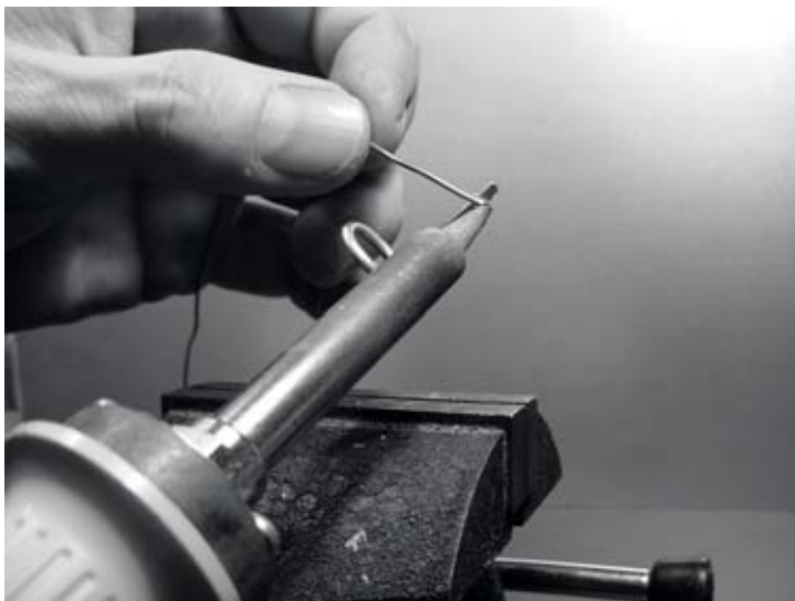
Figura 4.25: Adicione um pouco de solda ao final do fio, estanhando-o antes de soldá-lo.
